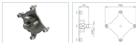
TTA3/4 (pour actionneurs munis d'une tête creuse)
